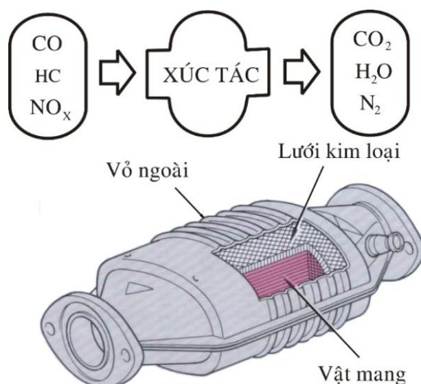
Hình 3. 8. Thiết bị xúc tác
